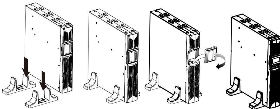
Rys. 1 Montaż Tower
